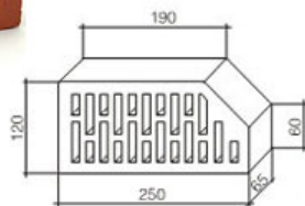
profil N-6
